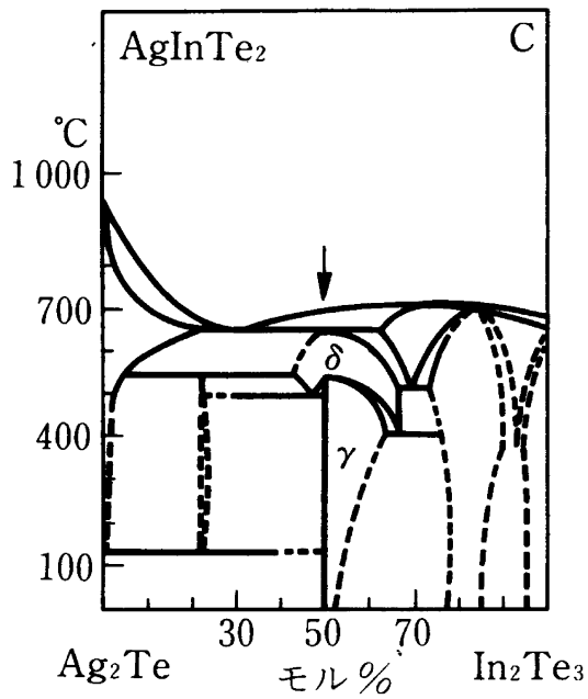
図 3.1: I-III-VI 2 族カルコパイライト型化合物の擬二元相図 [18]
