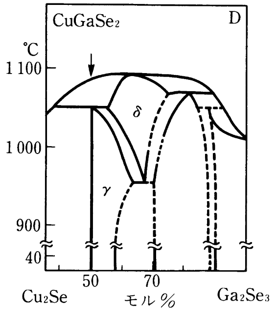
図 3.1: I-III-VI 2 族カルコパイライト型化合物の擬二元相図 [18]
