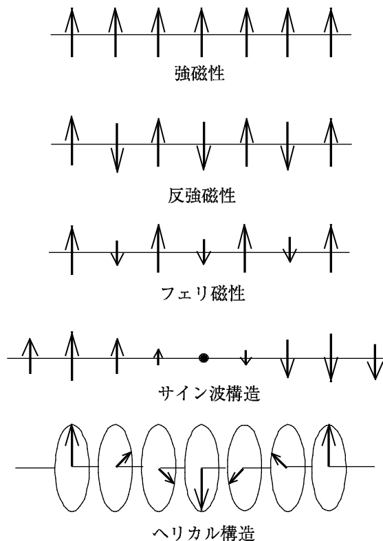
FIG. 1. いろいろな磁石の磁気構造。ここで矢印は結晶中で一方向に進んだ時の各磁性イオンでの磁化の大きさと向きを表す。磁石には、鉄のように磁化の向きが一方向に揃った強磁性体の他に、隣のイオンでは磁化の向きが反平行になっている反強磁性体、反強磁性体の特殊な場合で向きの異なる磁化の大きさの異なるフェリ磁性体、また場所ごとに磁化の大きさが三角関数的に波打っているサイン波構造（スピン密度波）の磁性体、一方向に進んでいくとき磁化の向きが螺旋状に回転しているヘリカル構造の磁性体、等がある。サイン波構造は金属の磁性体（典型的な遷移電子磁性体）で現れることがあり、ヘリカル構造は絶縁体の磁性体で現れることがある。
